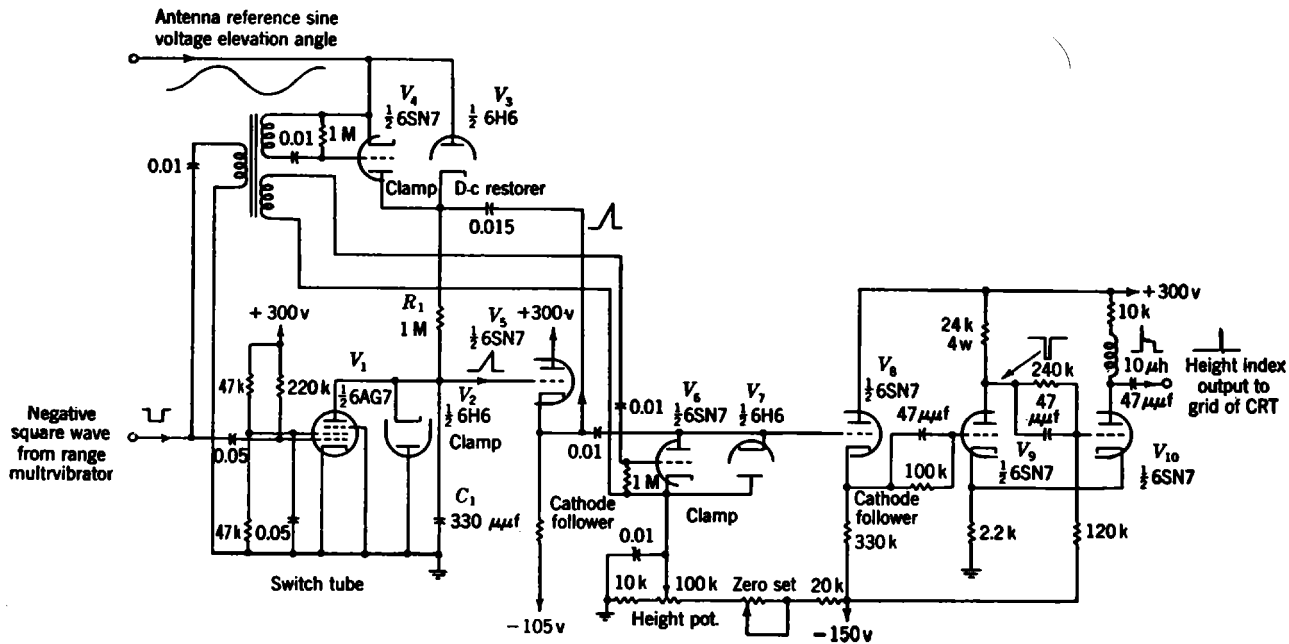
FIG. 6-18.—Height-index circuit.
